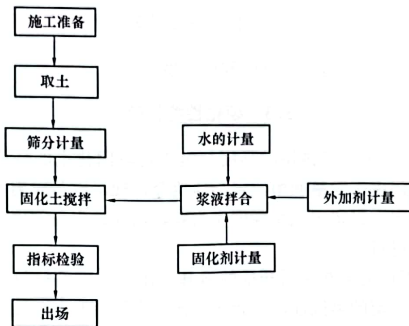
图 1 固化土的制备工艺流程
